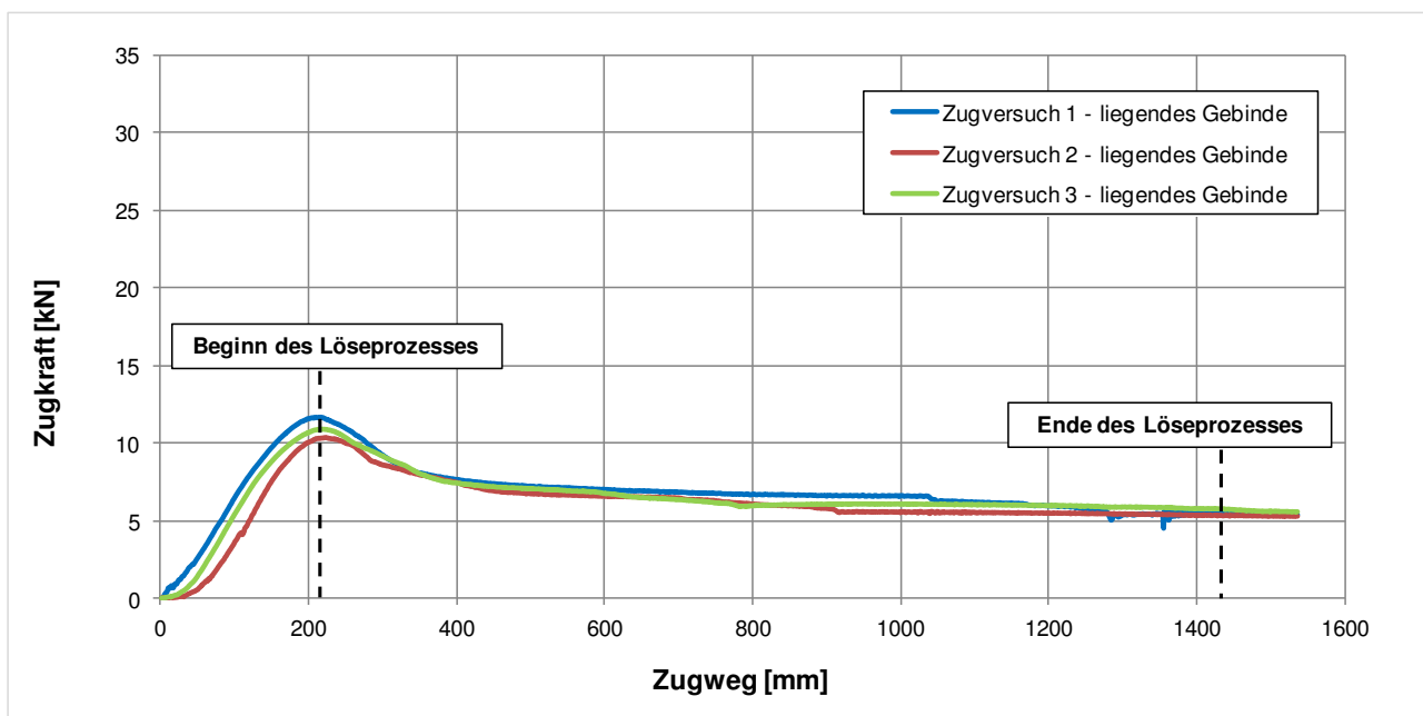
Abbildung 110: Zugkraftverlauf der liegend eingebrachten Gebinde mit Vakuumheber.
