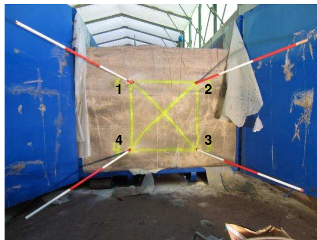
Abbildung 72: Lage und Winkel der Bohrlöcher im Steinsalzbetonblock.
