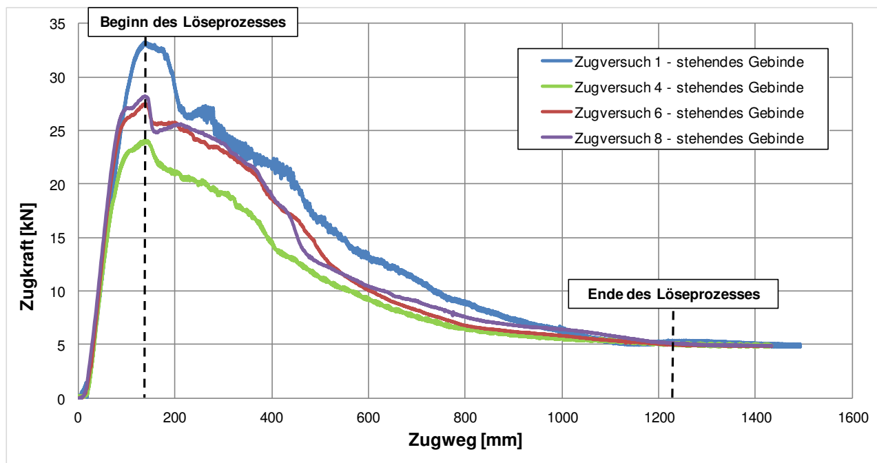
Abbildung 109: Zugkraftverlauf der stehend eingebrachten Gebinde mit Lasthaken.
