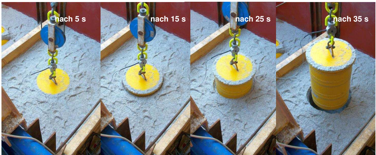
Abbildung 100: Fotostrecke beim Ziehen stehend eingebrachter Gebinde.
