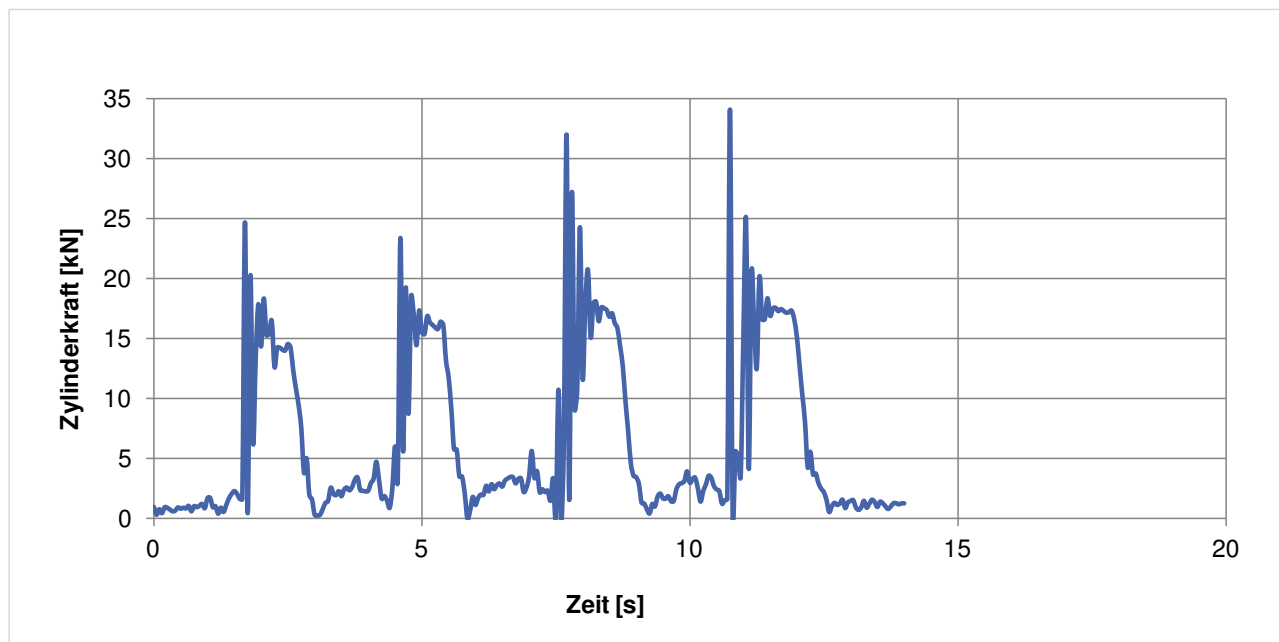
Abbildung 24: Scherversuch mit dem Baggerlöffel – Kraftverlauf im Löffelzylinder beim „Schlagen“.
