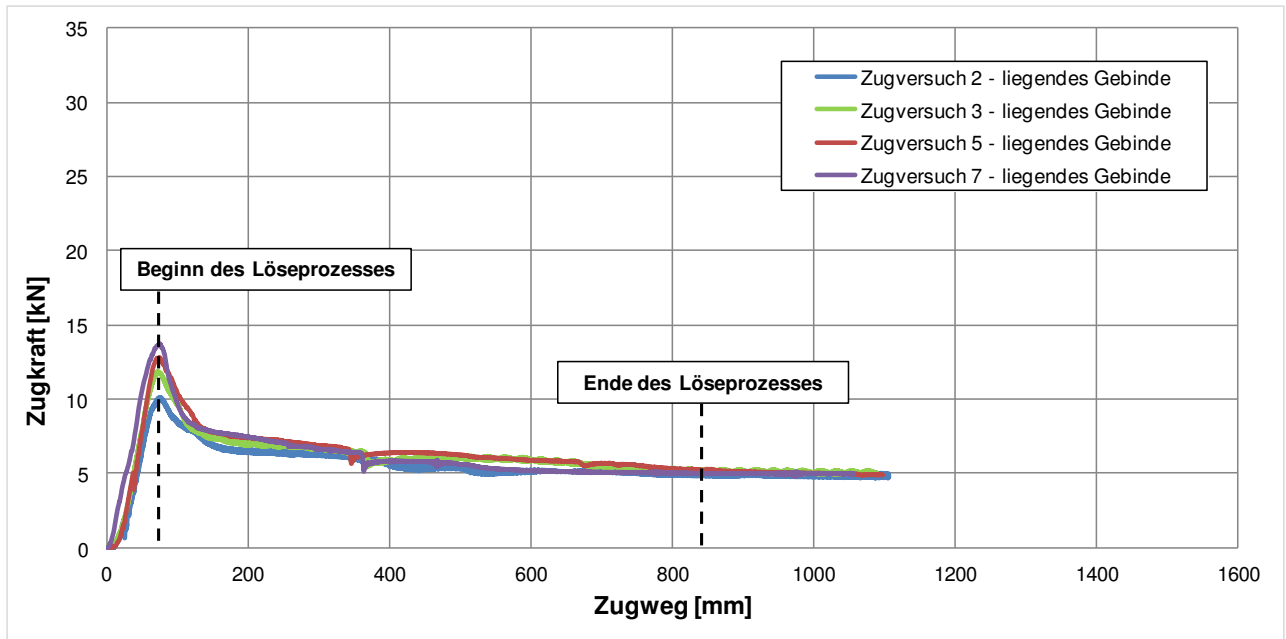
Abbildung 108: Zugkraftverlauf der liegend eingebrachten Gebinde mit Lasthaken.
