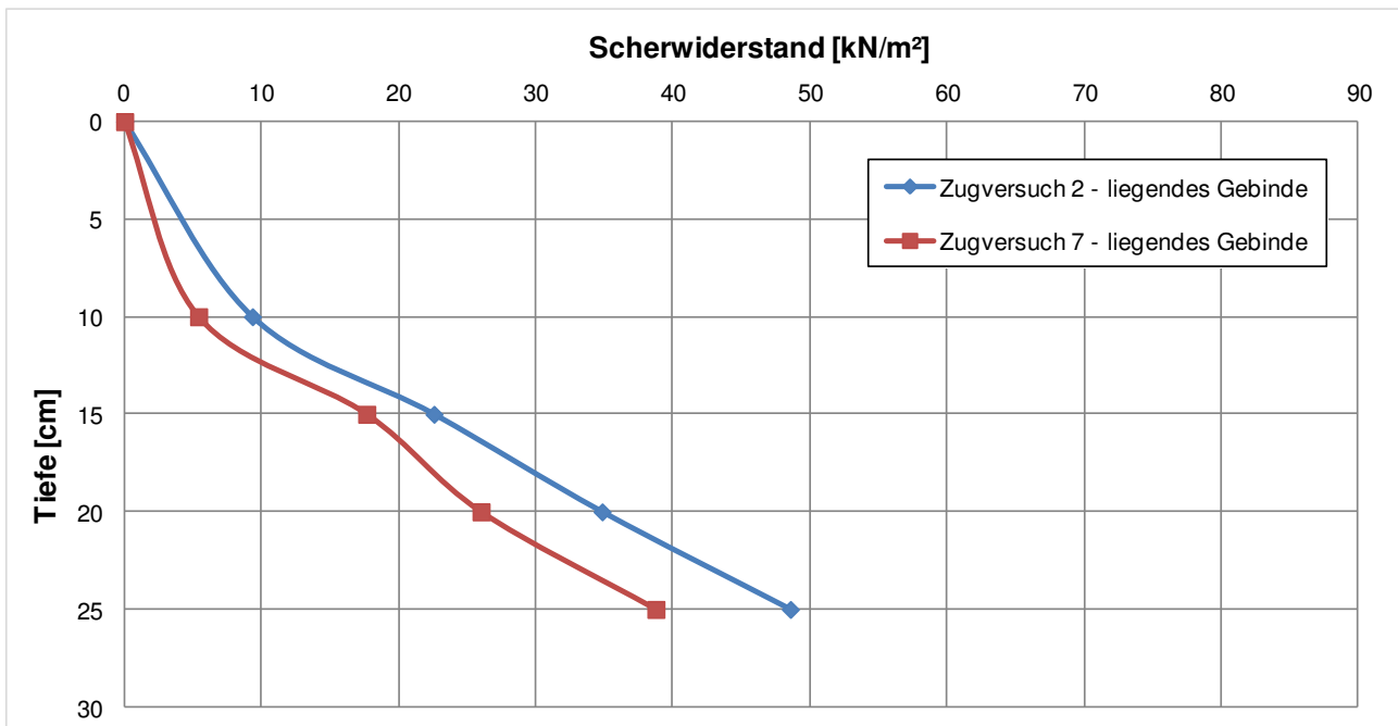
Abbildung 104: Ergebnisse der Flügelsondierung für Zugversuch 2 und Zugversuch 7.
