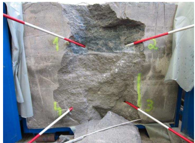
Abbildung 76: Abtragsergebnis des Spaltgeräts nach dem dritten Spaltvorgang.
