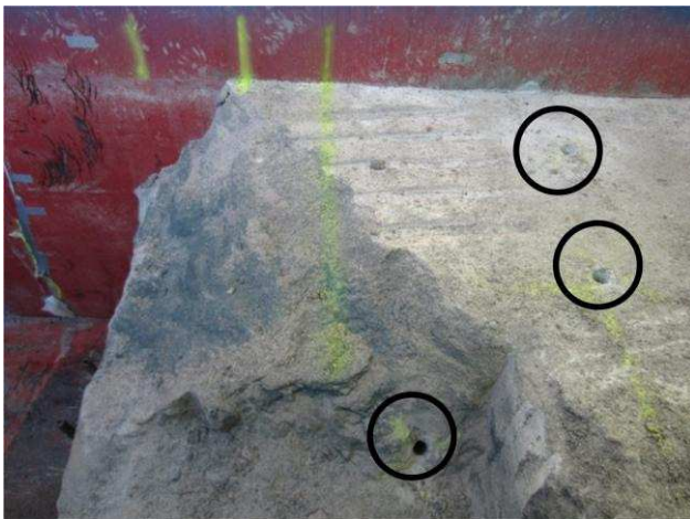
Abbildung 80: Für die Spaltversuche vorbereitete Bohrlöcher im Steinsalzbeton.
