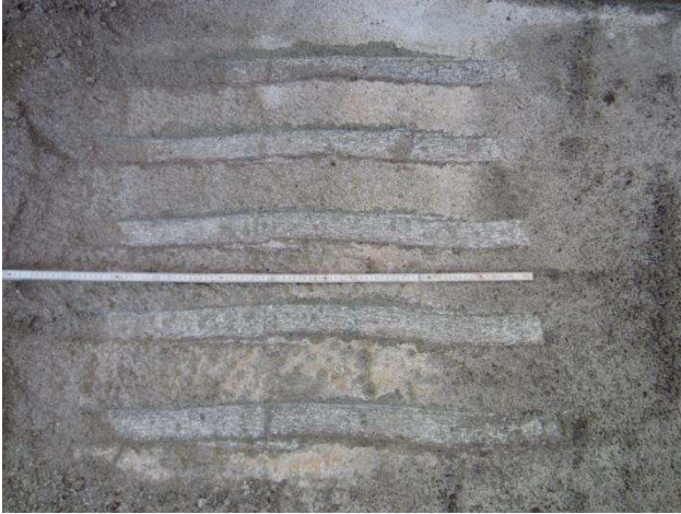
Abbildung 28: Schürfspur des Löffels im Steinsalzbeton.
