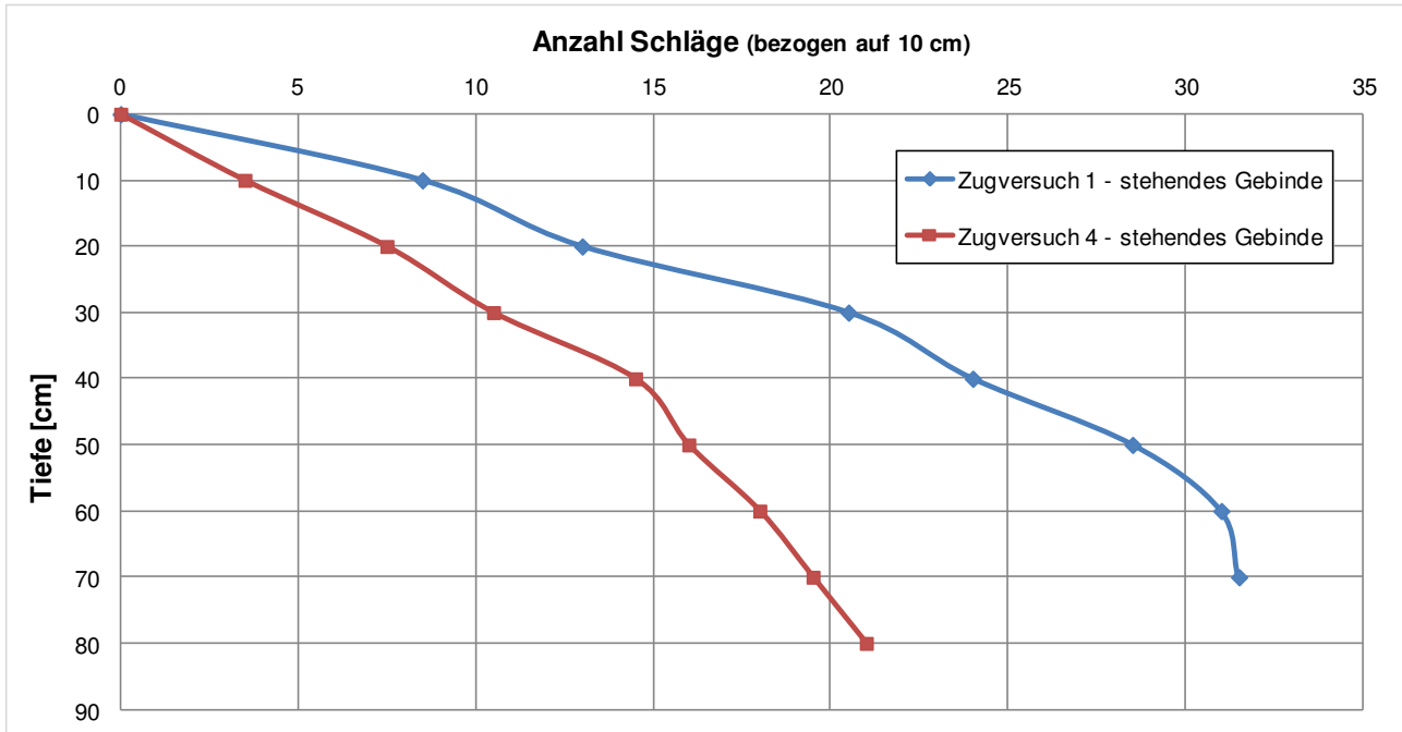
Abbildung 101: Ergebnisse der Rammsondierung für Zugversuch 1 und Zugversuch 4.
