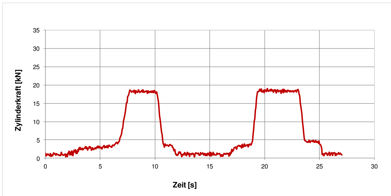
Abbildung 23: Scherversuch mit dem Baggerlöffel – Kraftverlauf im Löffelzylinder beim „Drücken“.
