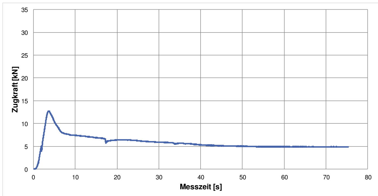
Abbildung 106: Zugkraftverlauf eines liegend eingebrachten Gebindes mit Lasthaken.
