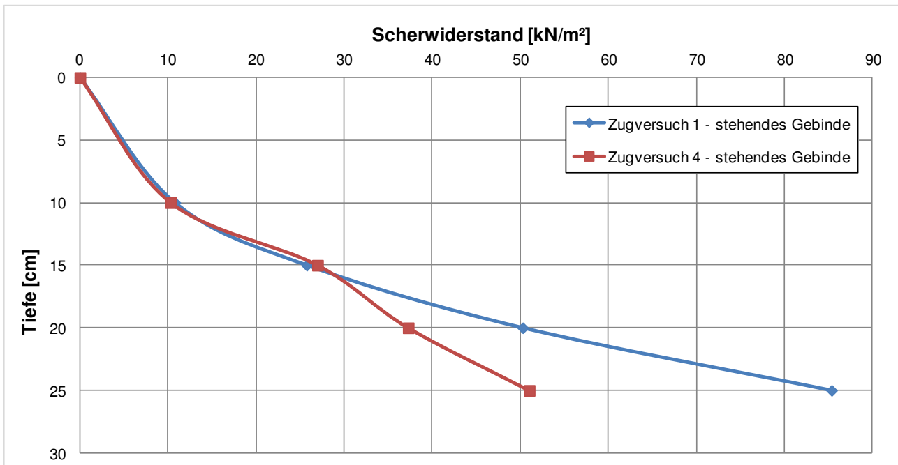
Abbildung 102: Ergebnisse der Flügelsondierung für Zugversuch 1 und Zugversuch 4.
