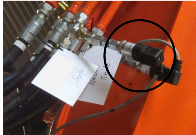
Abbildung 18: Druckmessumformer des Herstellers Hydac International GmbH vom Typ HDA 4745-A-600-000 am Trägergerät.
