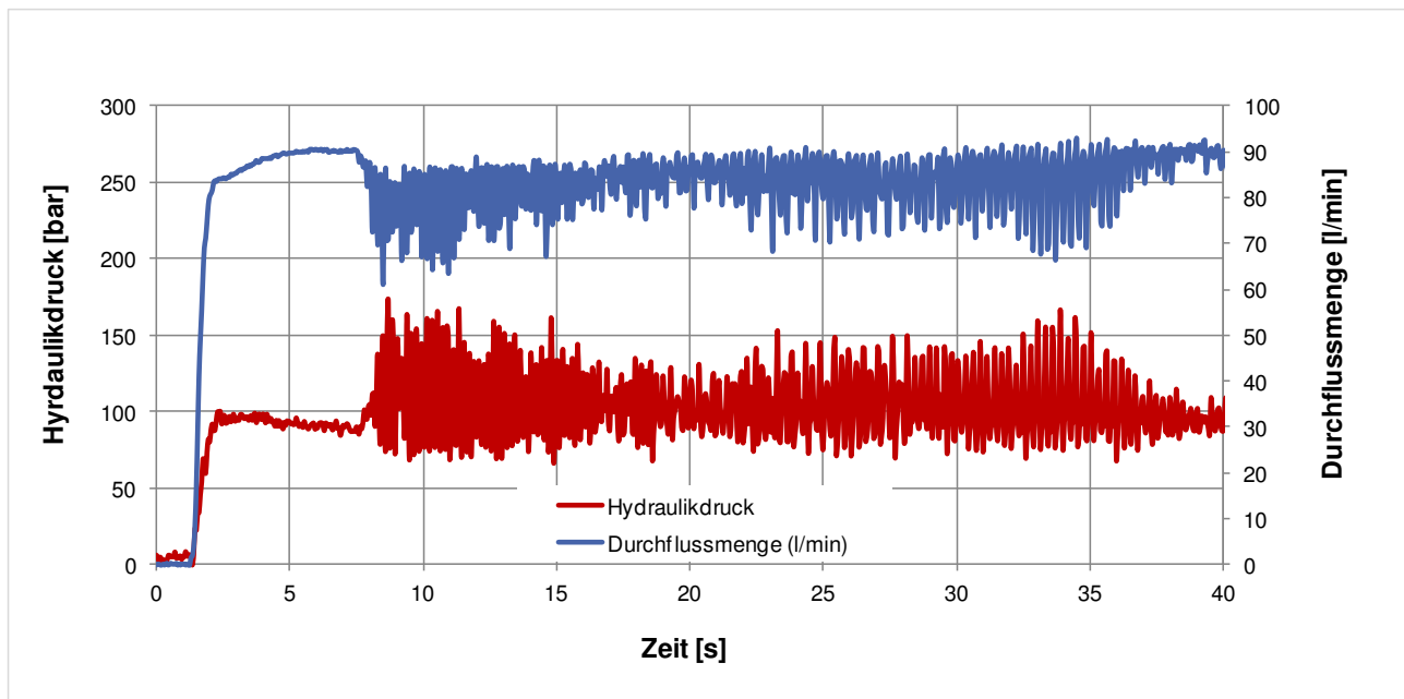
Abbildung 46: Durchflussmenge und Hydraulikdruck beim Fräsen in Steinsalzbeton.
