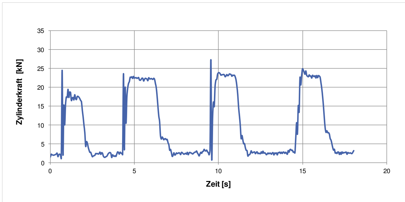
Abbildung 36: Scherversuch mit dem Reißzahn – Kraftverlauf im Löffelzylinder beim „Schlagen“.
