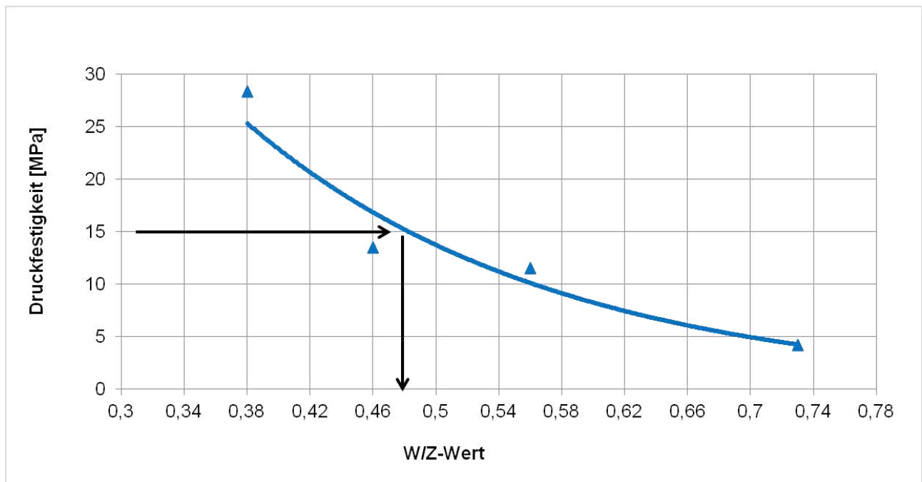
Abbildung 6: Regressionsanalyse zur Bestimmung des W/Z-Wertes für eine Festigkeit von ca. 15 MPa.
