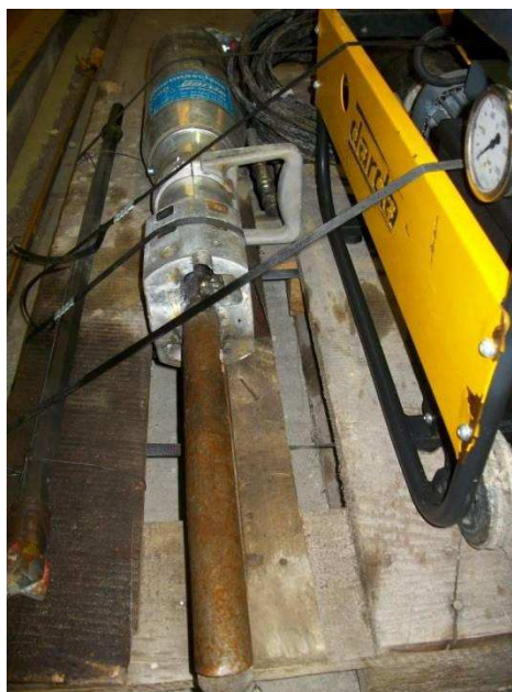
Abbildung 71: Eingesetztes Spaltgerät des Herstellers Darda GmbH vom Typ C 12 W mit Hydraulikaggregat.
