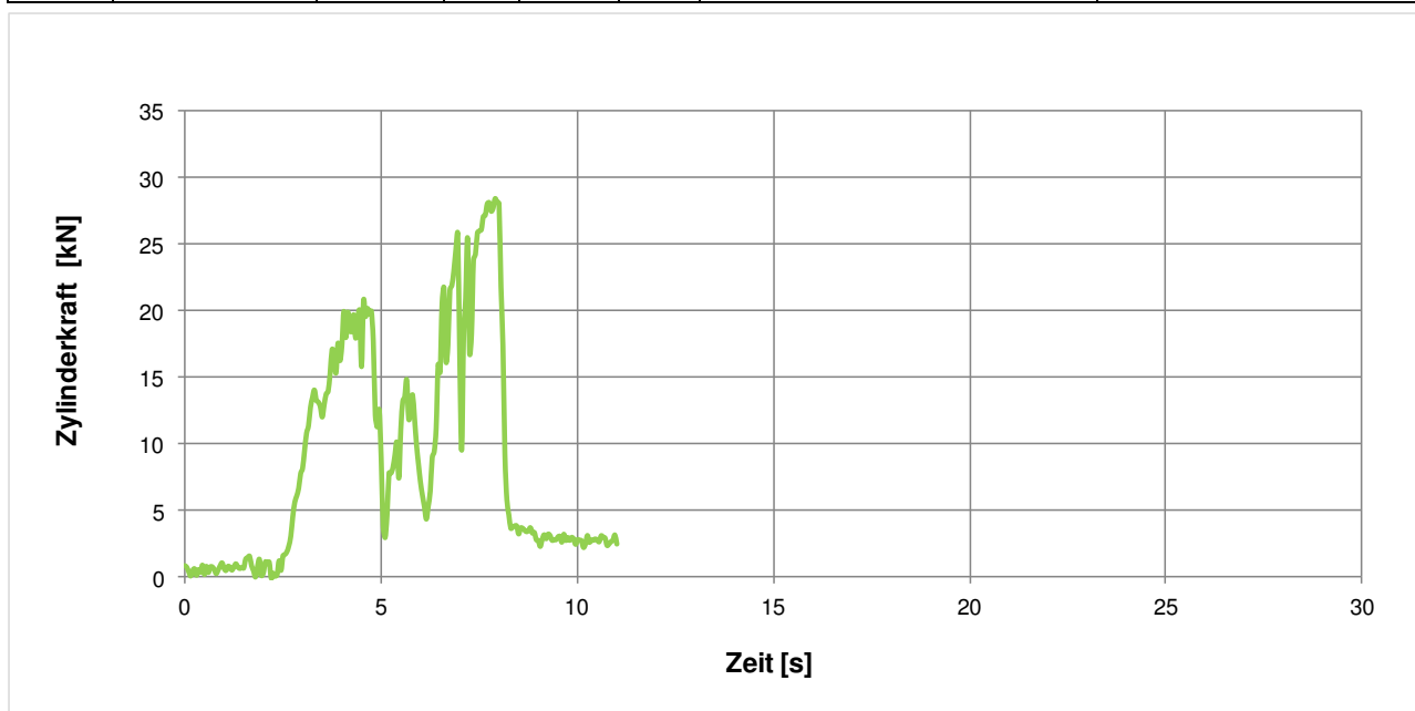
Abbildung 39: Schürfversuch mit Reißzahn – zeitlicher Kraftverlauf im Löffelzylinder.
