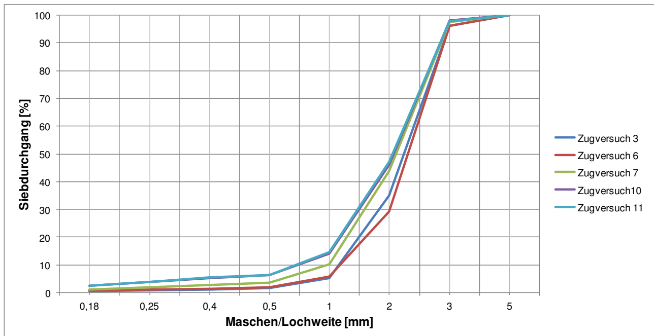
Abbildung 105: Siebanalyse der Salzmatrix zur Bestimmung der Korngrößenverteilung.
