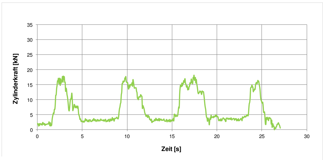
Abbildung 27: Schürfversuche mit dem Löffel – Kraftverlauf im Löffelzylinder beim Schürfen.
