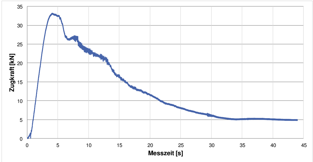
Abbildung 107: Zugkraftverlauf eines stehend eingebrachten Gebindes mit Lasthaken.
