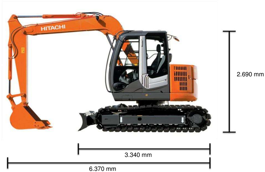
Abbildung 15: Trägergerät Hitachi ZX85US-3 [14].
