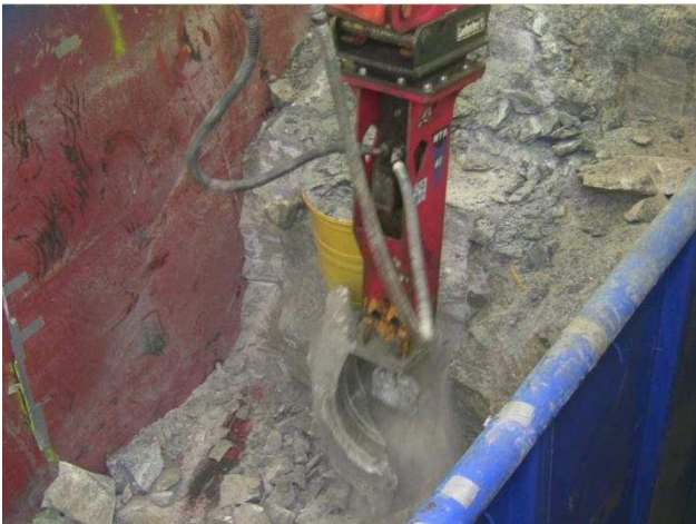
Abbildung 69: Hydraulikmeißel – „Abschälen“ des Steinsalzbetons vom eingeschlossenen Gebinde.
