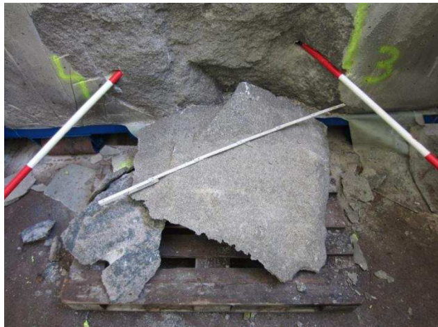
Abbildung 77: Durch den dritten Spaltvorgang erzeugtes Bruchstück aus dem Steinsalzbeton.
