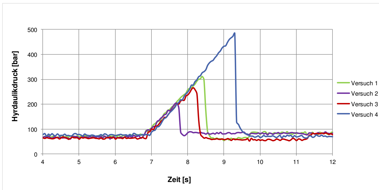
Abbildung 79: Spaltversuche 1 bis 4 – Hydraulikdruck in Abhängigkeit der Zeit.
