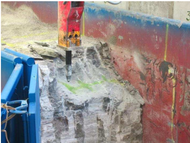
Abbildung 65: Ansatzpunkte im Steinsalzbetonblock für Test mit Spitzmeißel.
