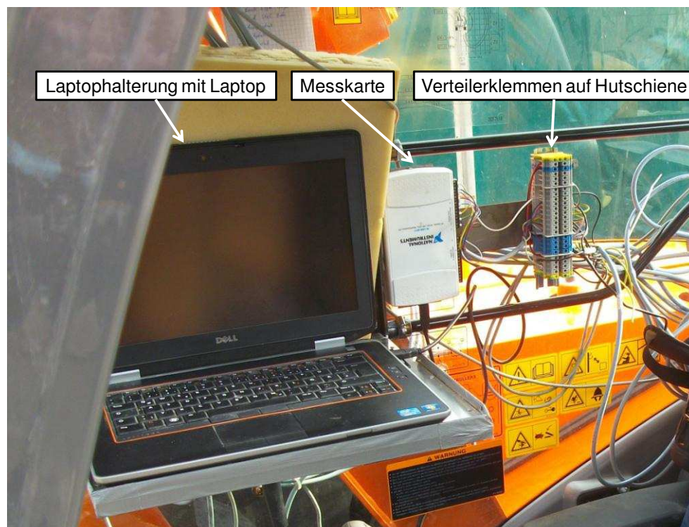
Abbildung 17: Eingesetzte Messtechnik am Trägergerät.
