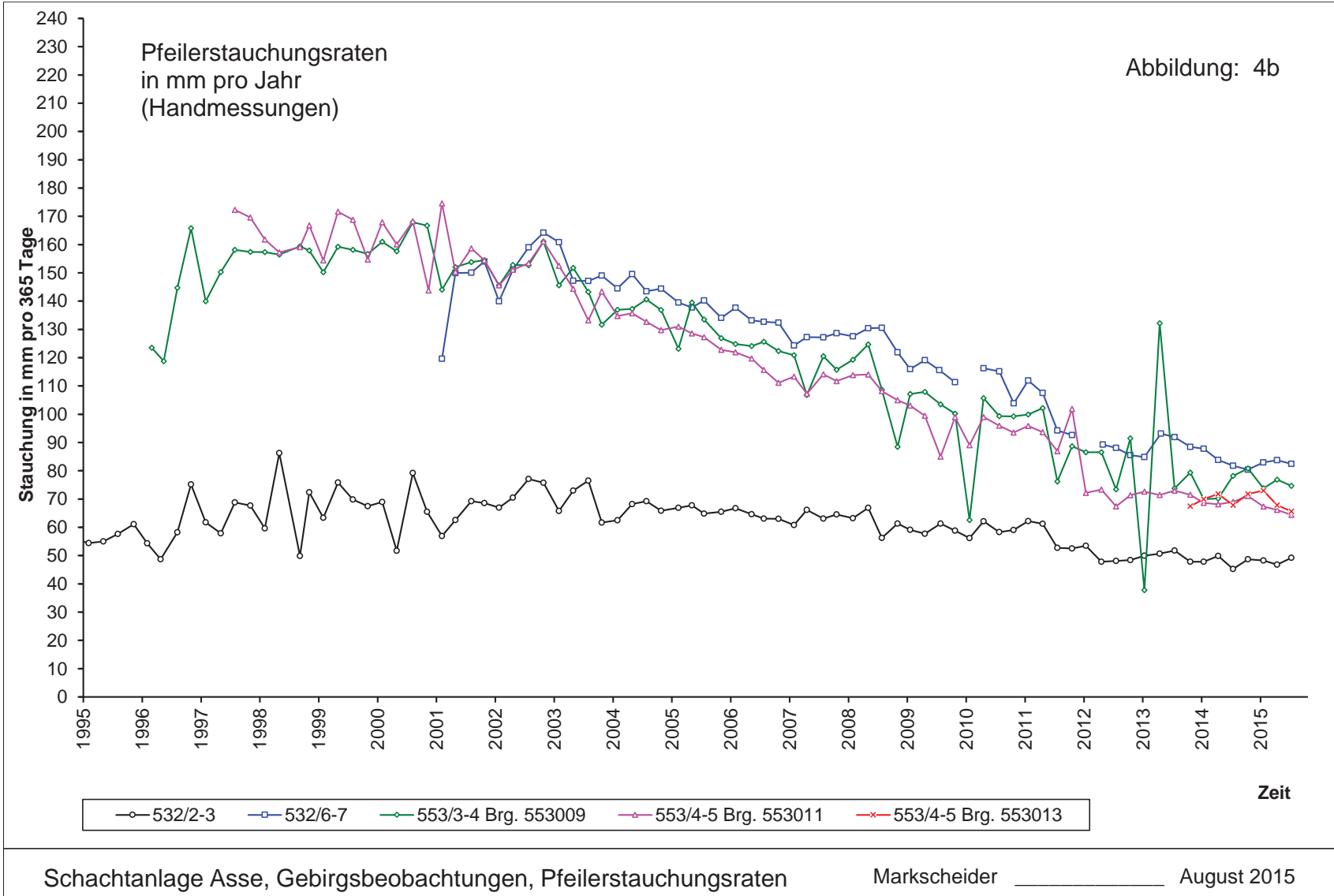
Abbildung 4b: Pfeilerstauchungsraten 532- und 553-m-Sohle [mm/a]
