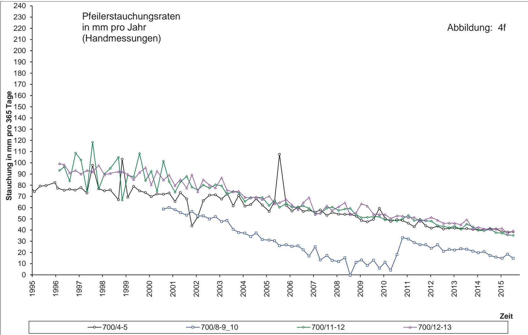
Abbildung 4f: Pfeilerstauchungsraten 700-m-Sohle [mm/a]
