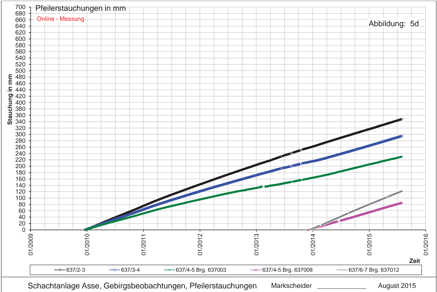
Abbildung 5d: Pfeilerstauchungen [mm] der Extensometer auf der 637-m-Sohle (elektronische Messwerte)
