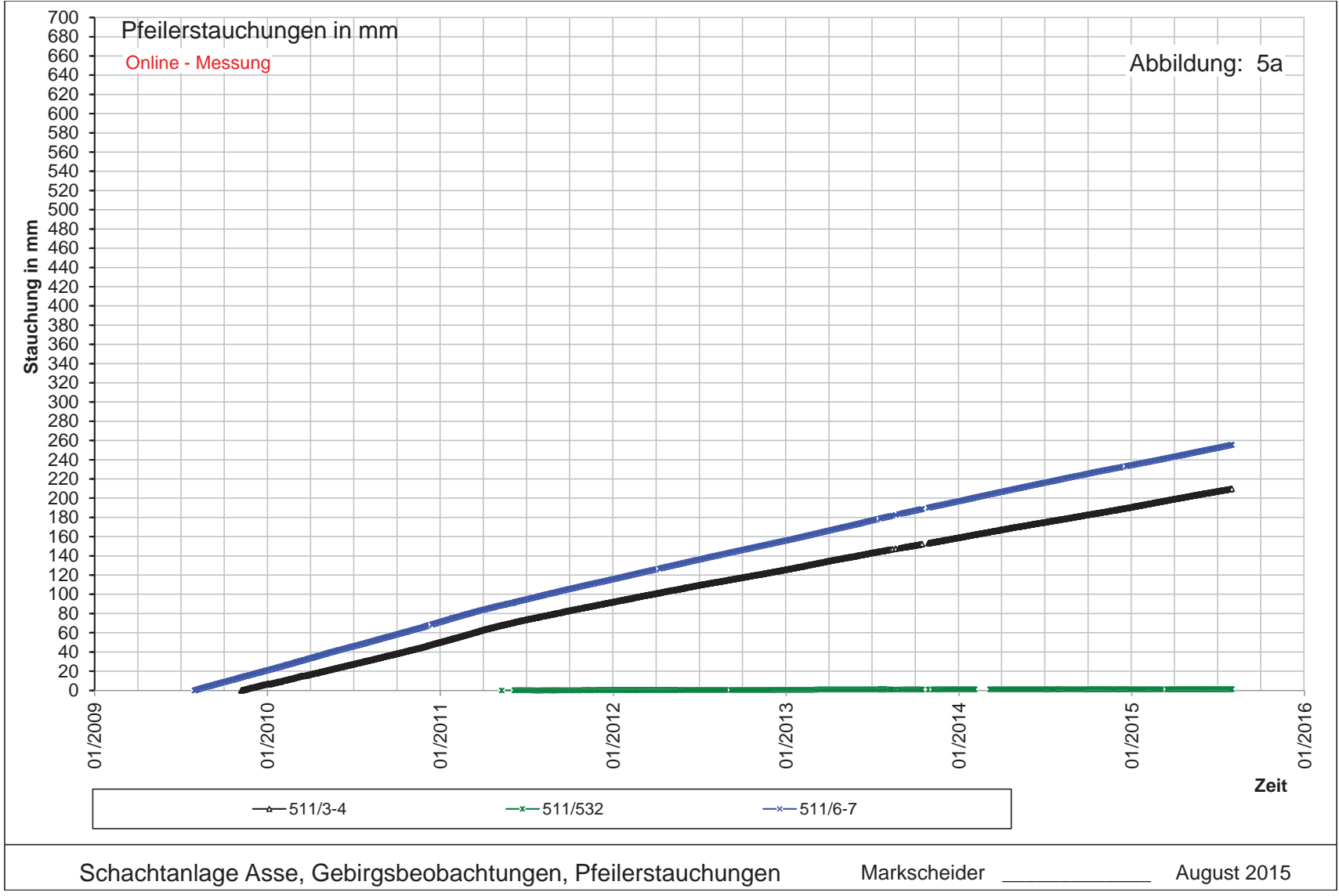
Abbildung 5a: Pfeilerstauchungen [mm] der Extensometer auf der 511-m-Sohle (elektronische Messwerte)
