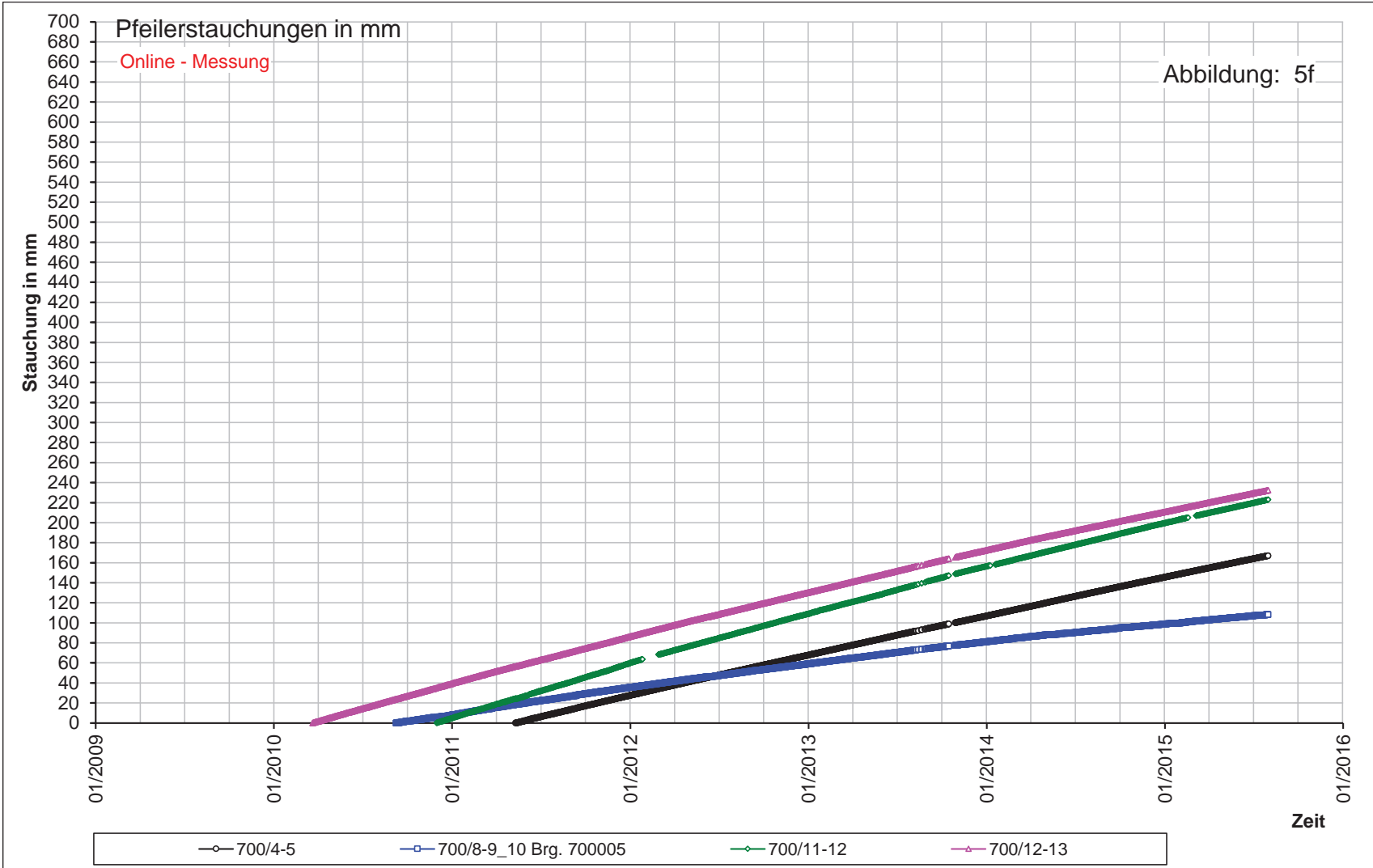
Abbildung 5f: Pfeilerstauchungen [mm] der Extensometer auf der 700-m-Sohle (elektronische Messwerte)
