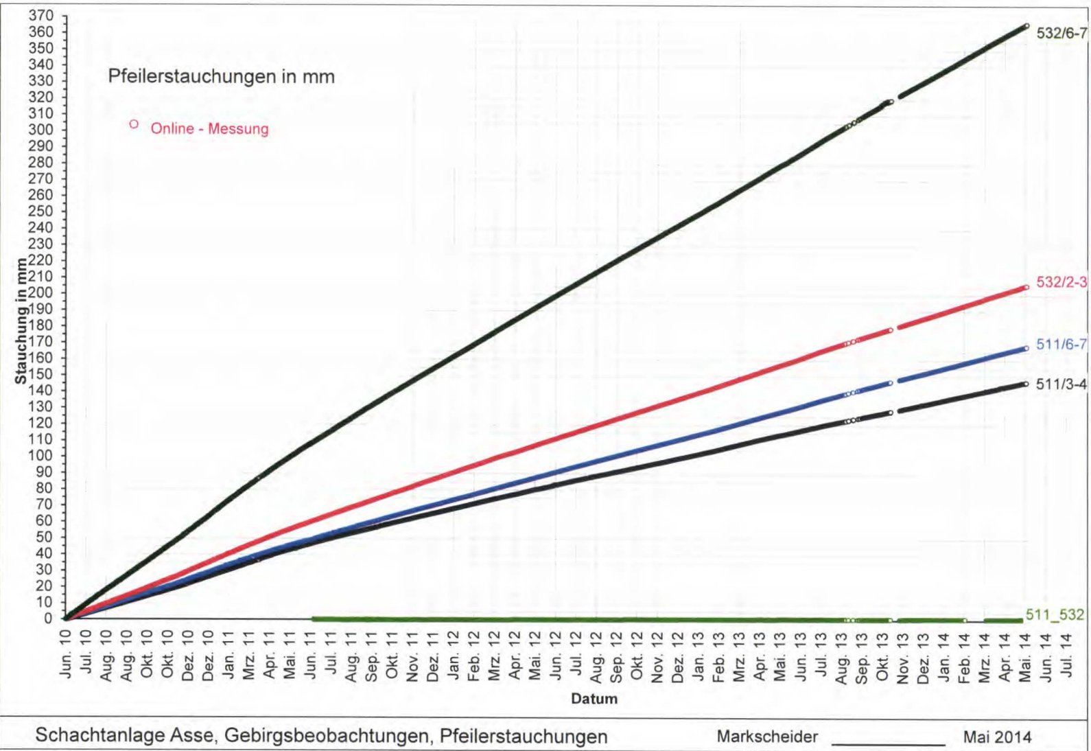
Abbildung 5a: Elektronische Messwerte der Extensometer auf der 511 - und 532-m-Sohle
