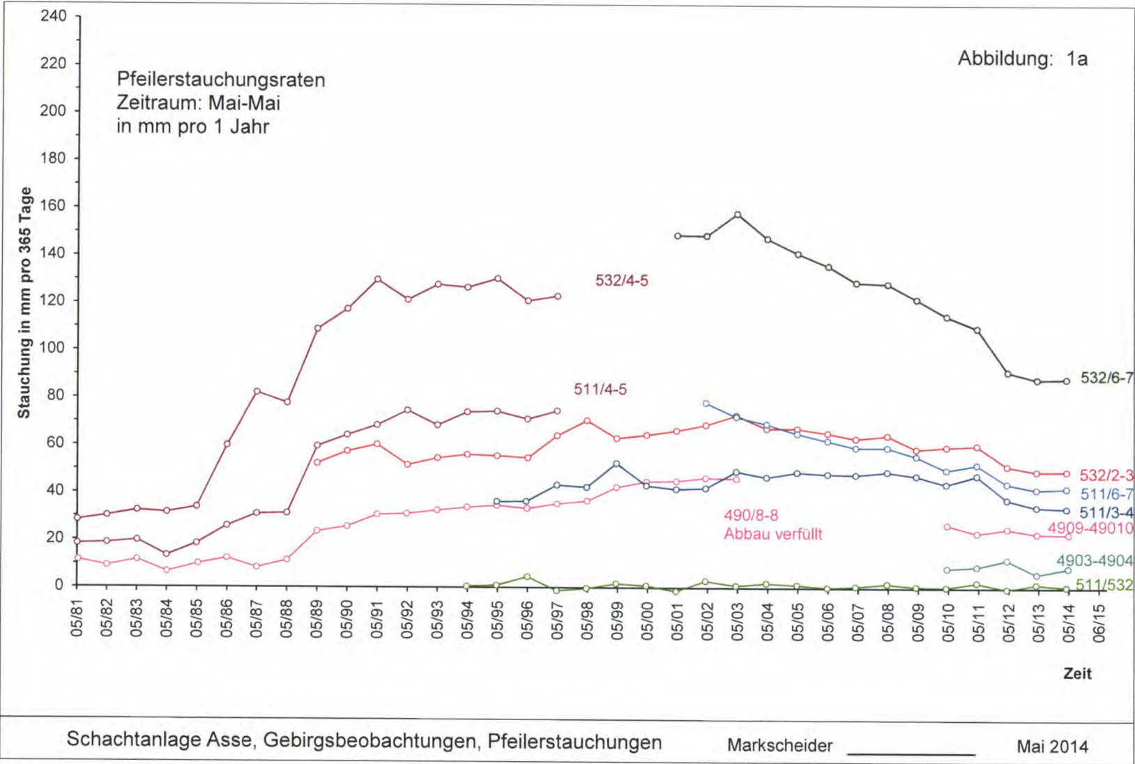
Abbildung 1a: Absolute Pfeilerstauchung [mm] zwischen der 511- und 532-m-Sohle
