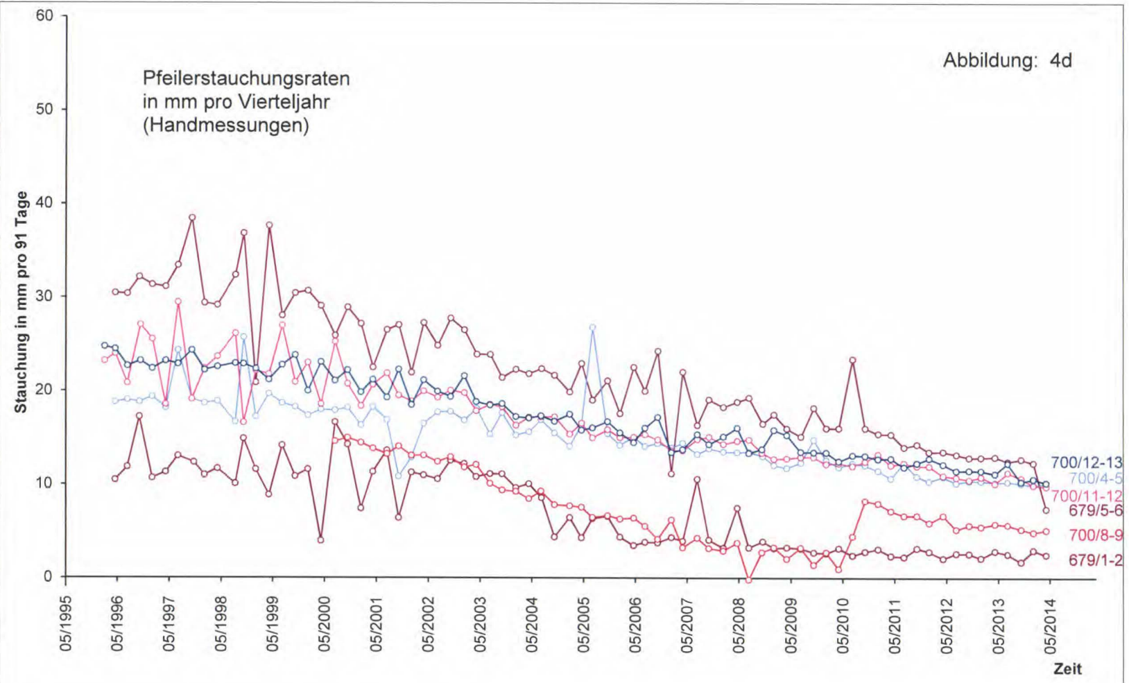
Abbildung 4d: Pfeilerstauchungsraten 679- und 700-m-Sohle [mm/91 Tage]
