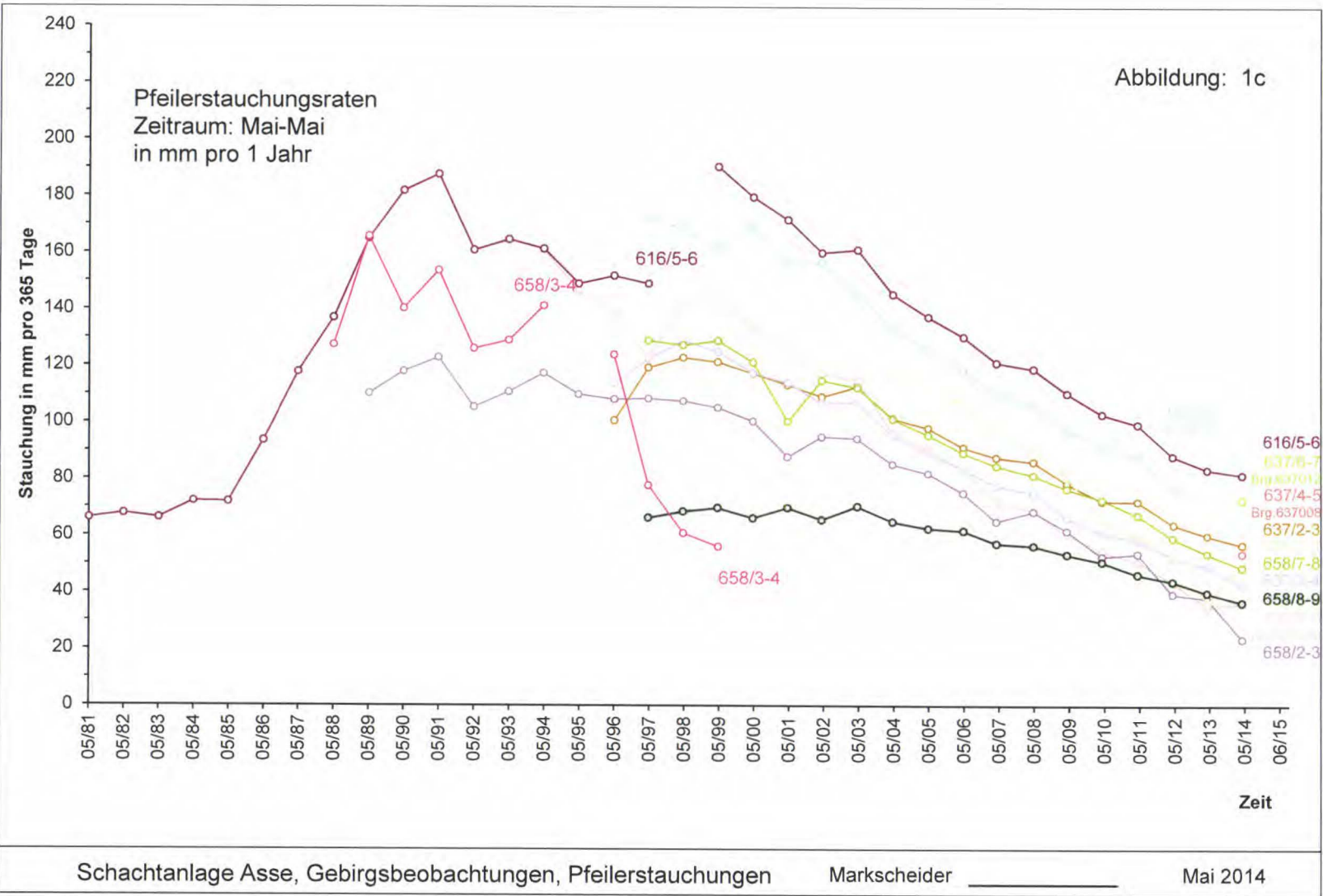
Abbildung 1c: Absolute Pfeilerstauchung [mm] zwischen der 616- und 658-m-Sohle
