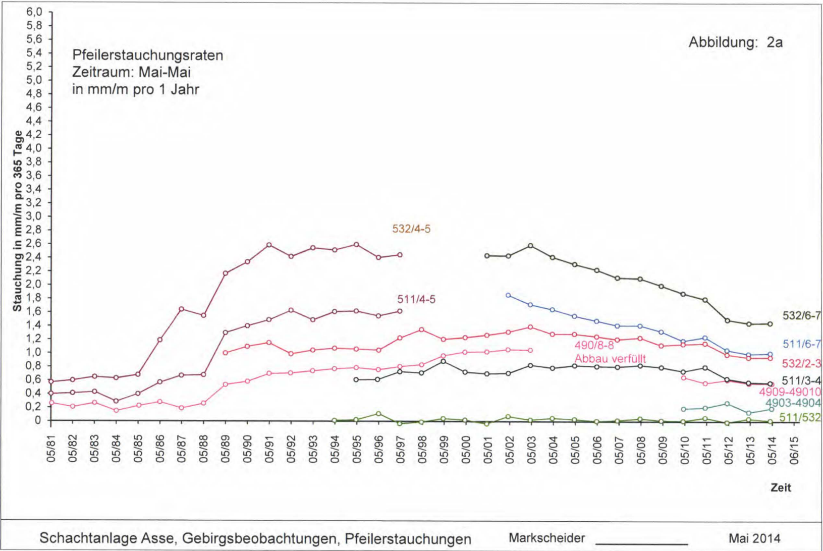
Abbildung 2a: Pfeilerstauchungsraten 511- und 532-m-Sohle [mm/(m*a)]
