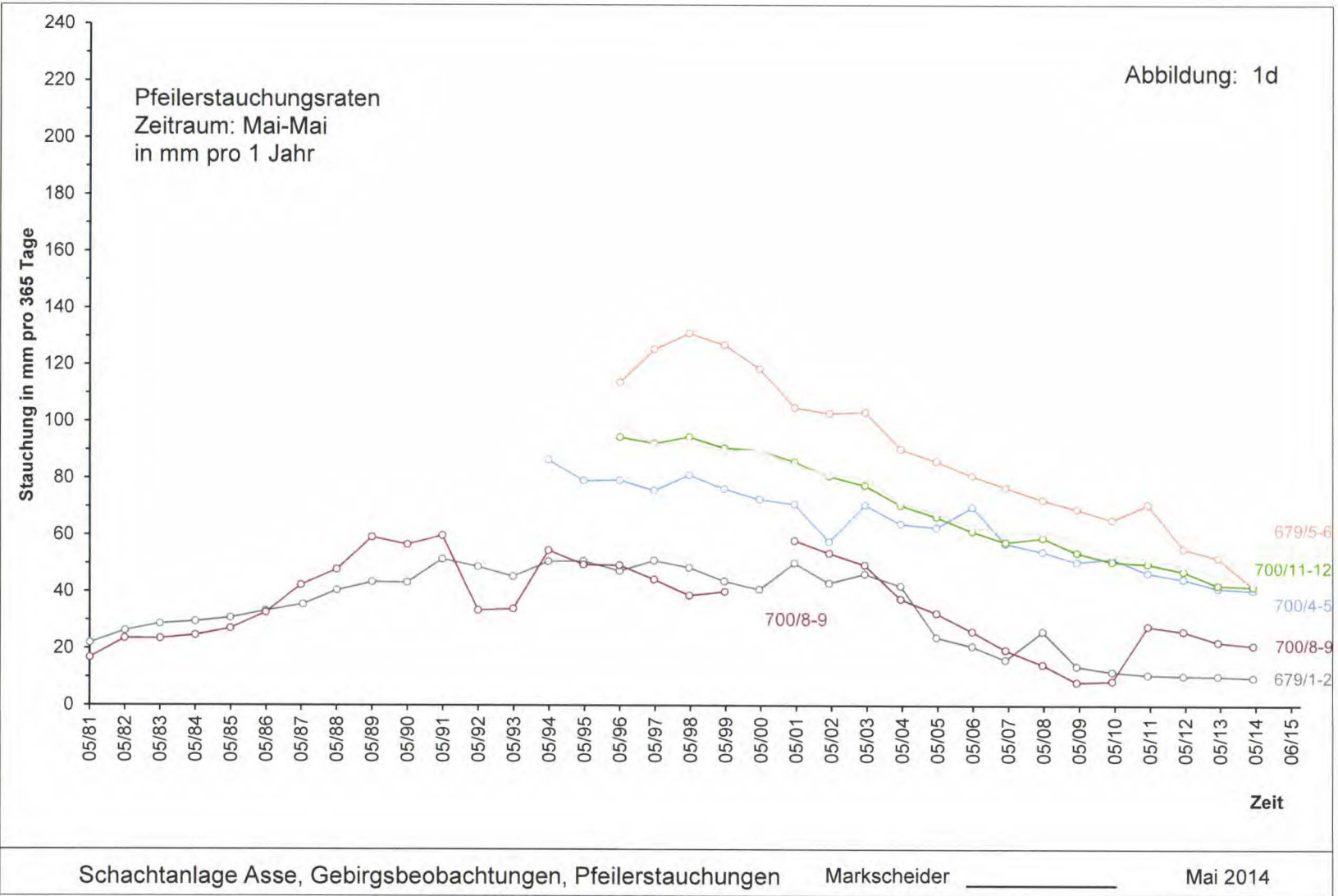
Abbildung 1d: Absolute Pfeilerstauchung [mm] zwischen der 679- und 700-m-Sohle
