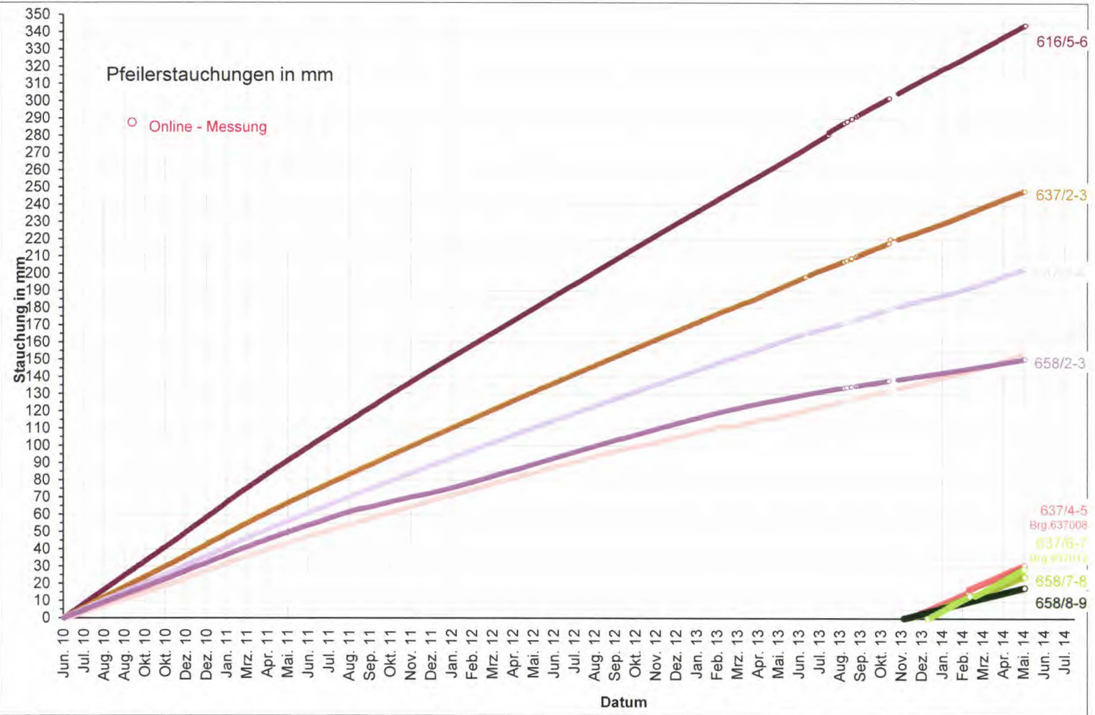
Abbildung 5c: Elektronische Messwerte der Extensometer auf der 616- bis 658-n-Sohle
